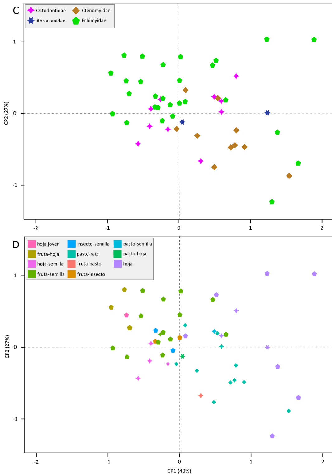
Figura S5.1: Proyección de las especies de Erethizontoidea (triángulos), Caviioidea (círculos) y Chinchilloidea (cuadrados) (A y B) y de Octodontoidea (C y D) en los dos primeros componentes del ACP. Cada punto representa el centroide de una especie. A. Los colores indican las familias: Erethizontidae (triángulos verdes), Cuniculidae (círculo verde claro), Dasyproctidae (círculos naranjas), Caviidae (círculos rojos), Dinomyidae (cuadrado violeta),
